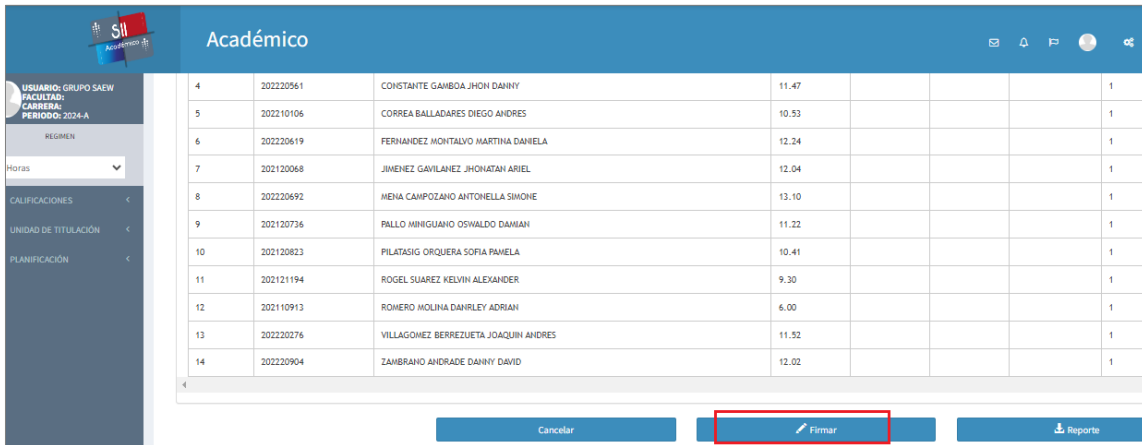
Figura 9: Botón Firmar
